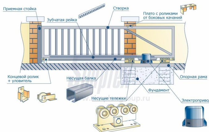
Конструкция сдвижных ворот
